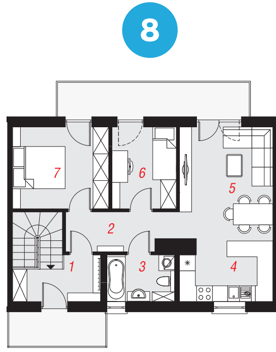
PIĘTRO
